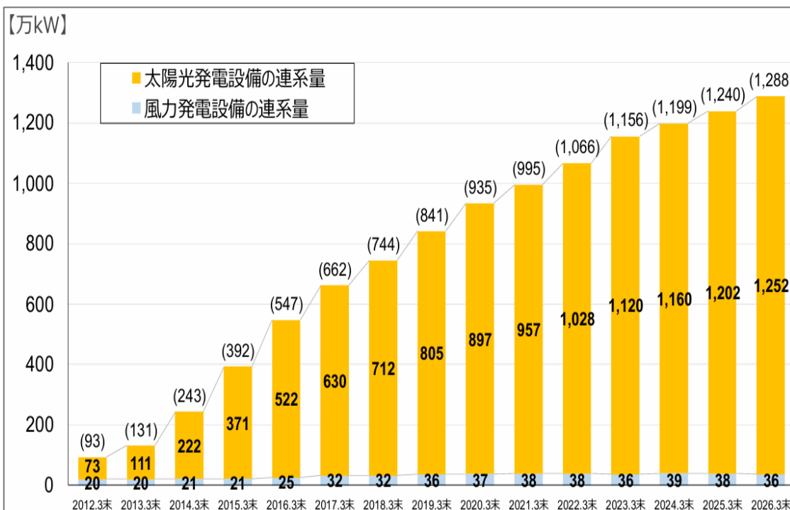
【中部エリアにおける太陽光・風力発電設備の連系量の推移】
