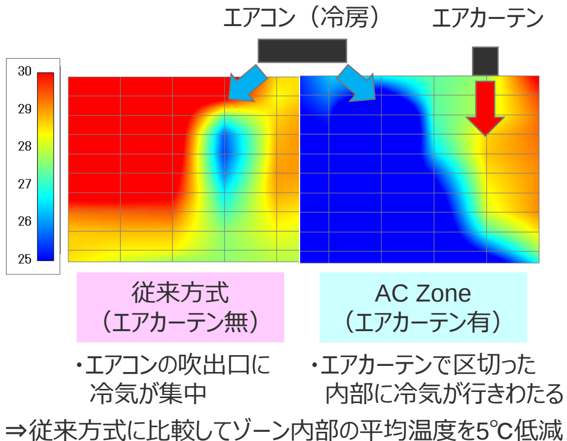
【ゾーン内部の温度分布】
