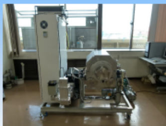
マイクロ波併用粉体加熱乾燥装置
